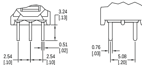
C - DPDT
